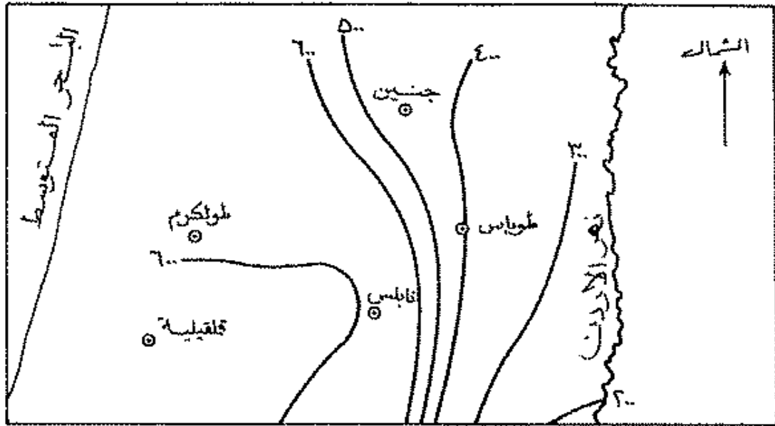
شكل (٥) معدل الأمطار السنوي (ملم) للفترة ١٩٣١ - ١٩٦٠
