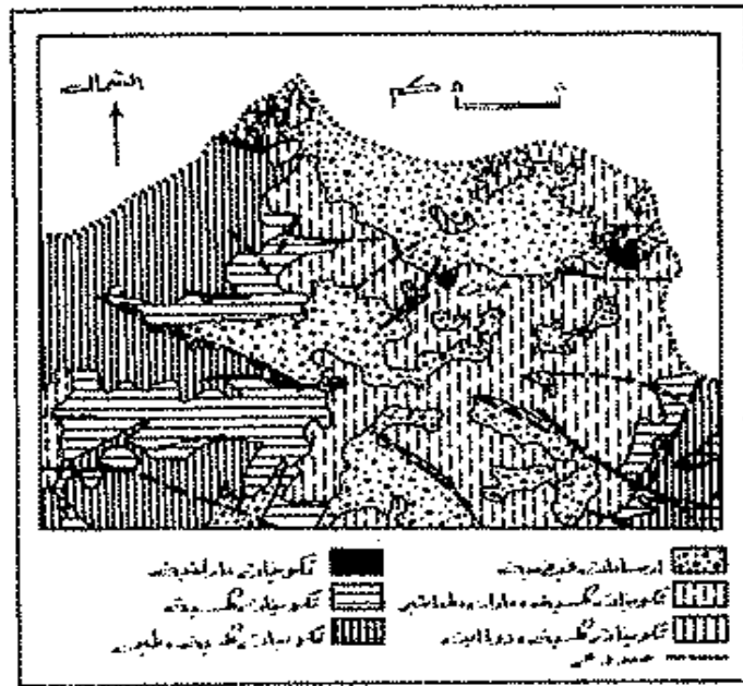
شكل (٣) خارطة جيولوجية لمنطقة جنين
