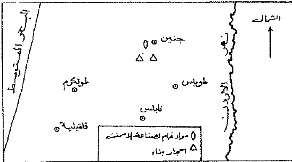
شكل (٤) الثروة المعدنية في منطقة جنين
